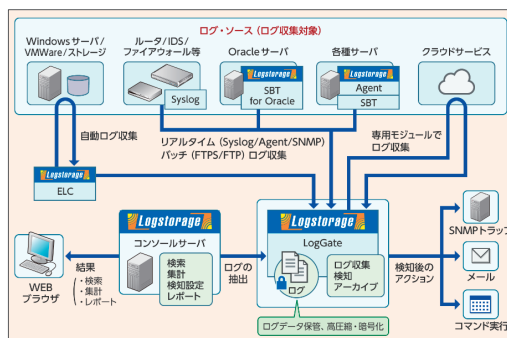
<Logstorage システム構成>
